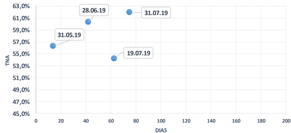
LECAP - CURVA DE RENDIMIENTOS
